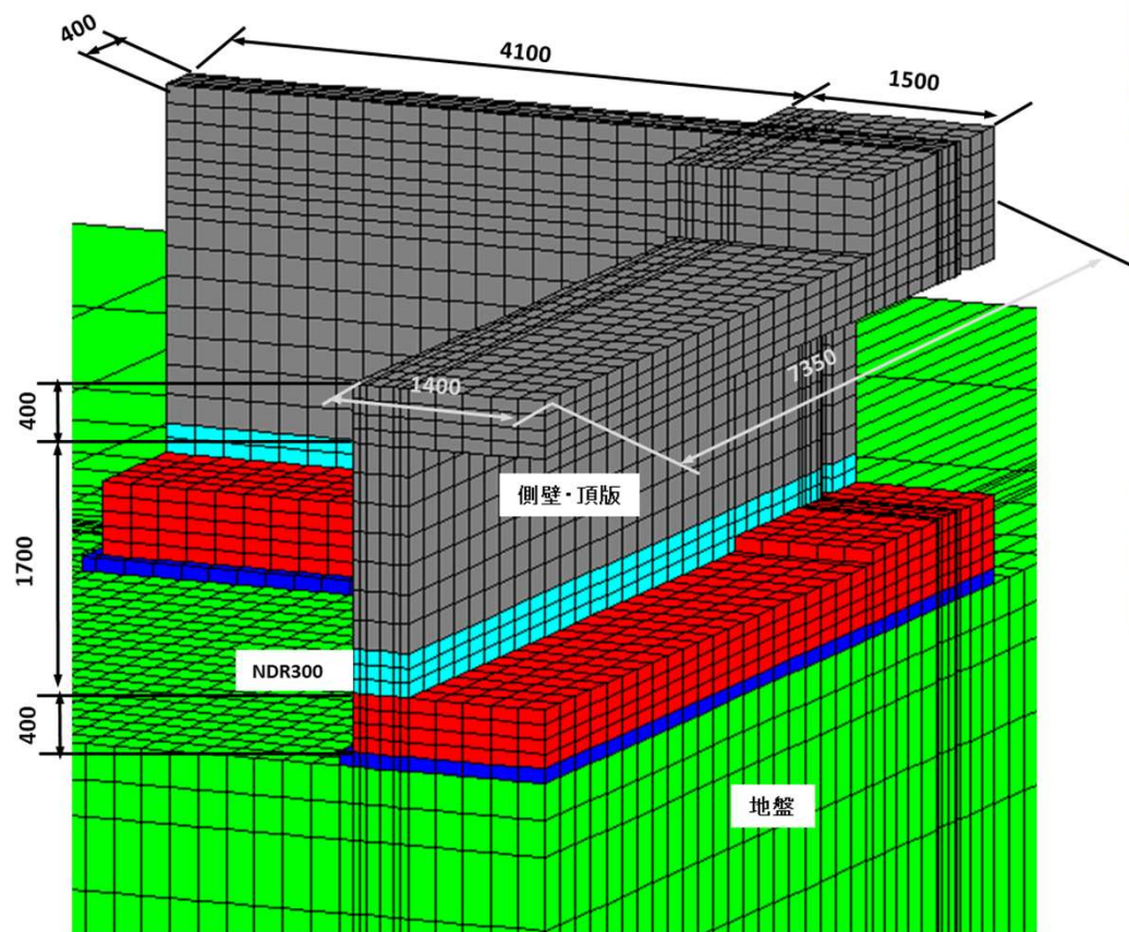
解析: 1/2対象モデル
