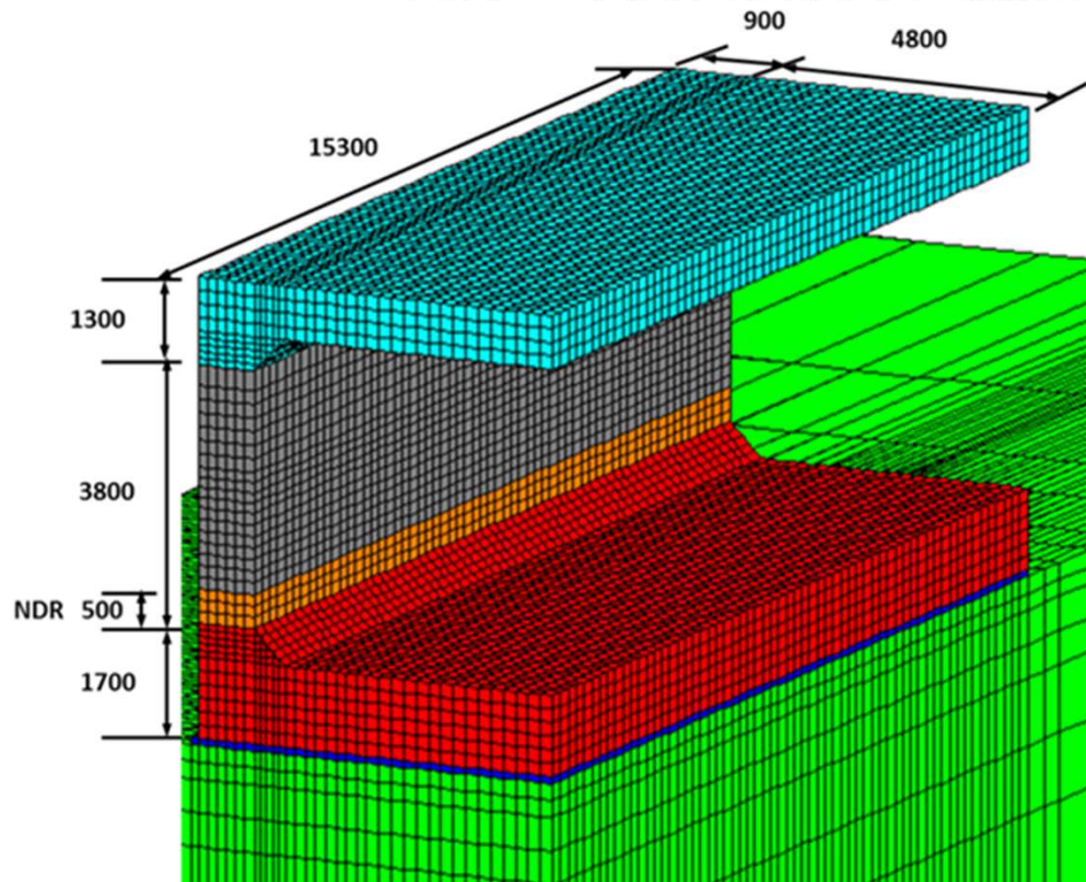
解析: 1/4対象モデル
