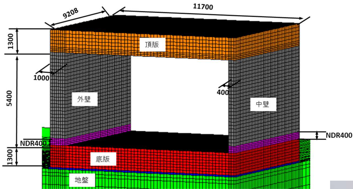
解析: 1/4対象モデル
