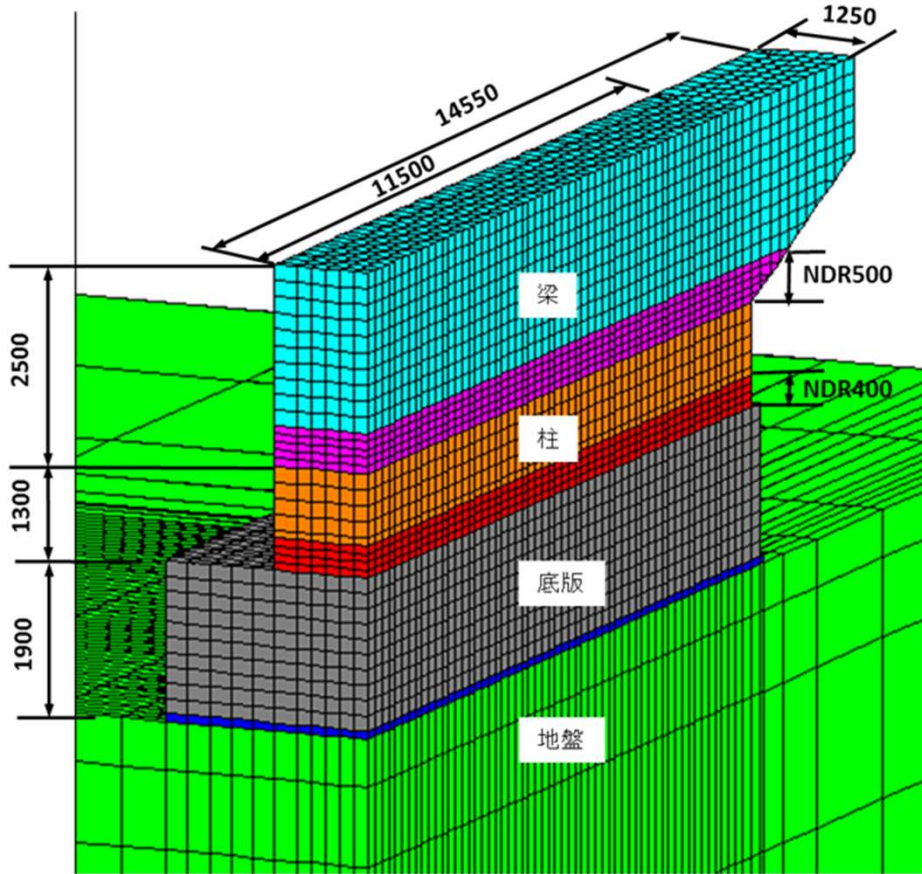
解析: 1/4対象モデル
