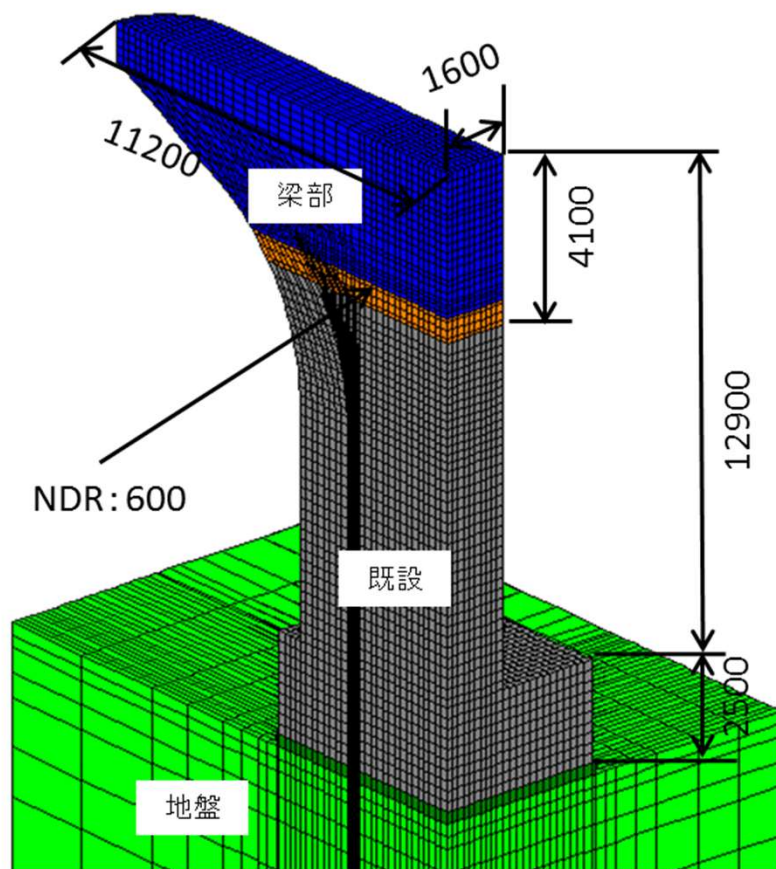
解析: 1/4対象モデル
