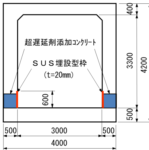
図-3 函渠工の断面図
