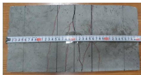
写真-4 曲げひび割れの分散状況
