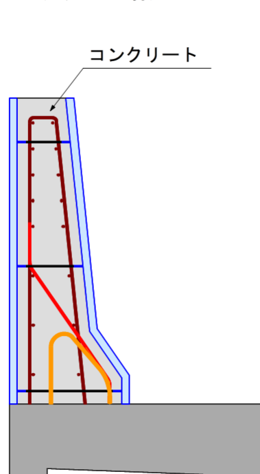
③コンクリートの打込み
