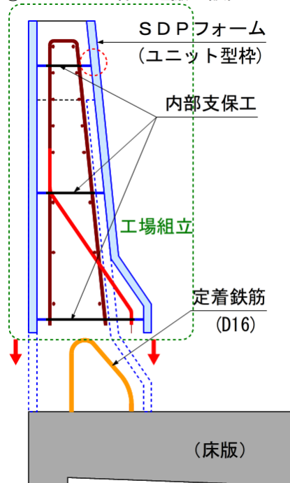
①ユニット型枠の運搬・設置
