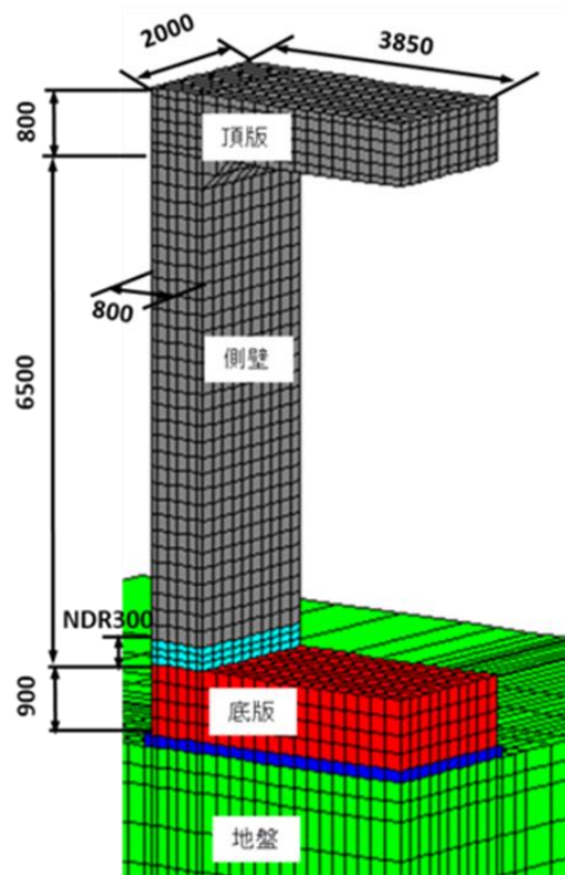
解析：1/4対象モデル
