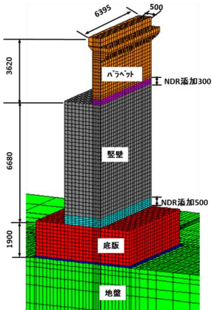
解析: 1/2対象モデル
