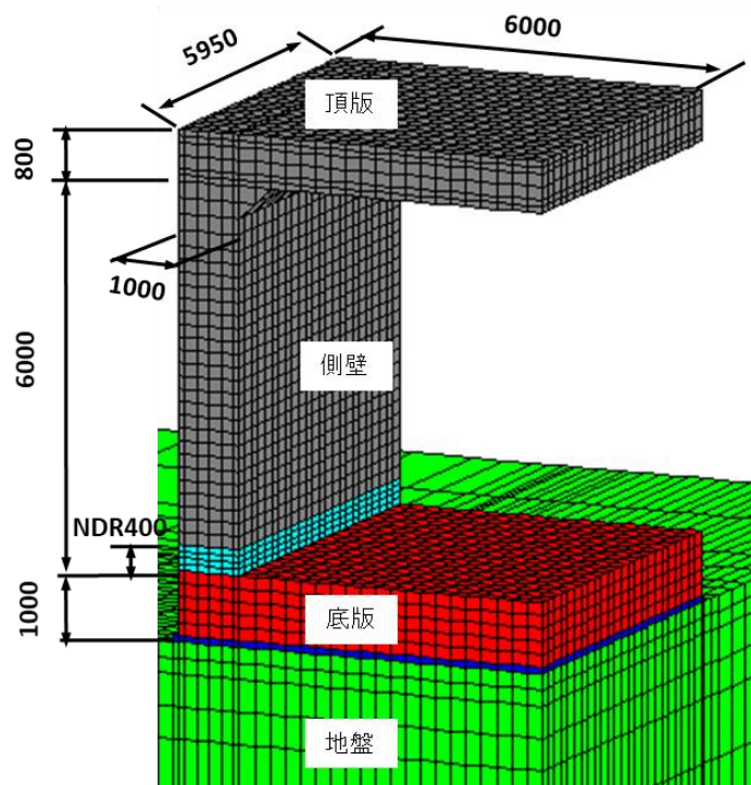
解析：1/4対象モデル
