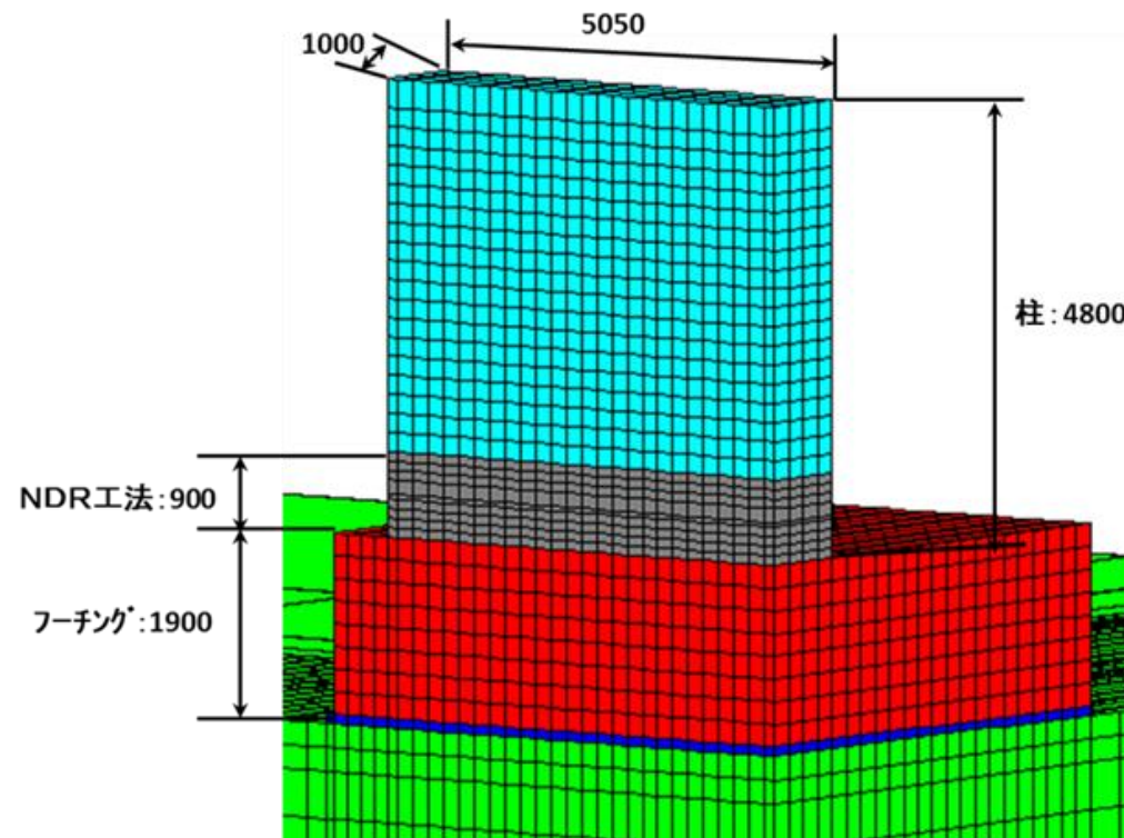
解析: 1/4対象モデル
