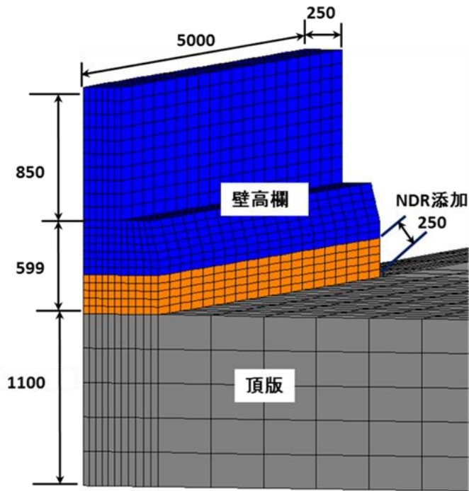
解析: 1/2対象モデル
