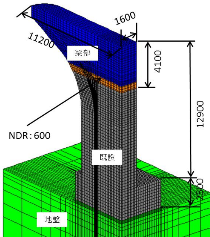
解析: 1/4対象モデル
