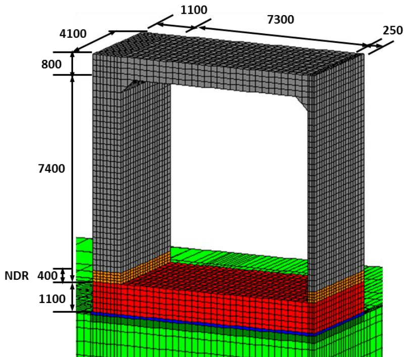
解析: 1/4対象モデル
