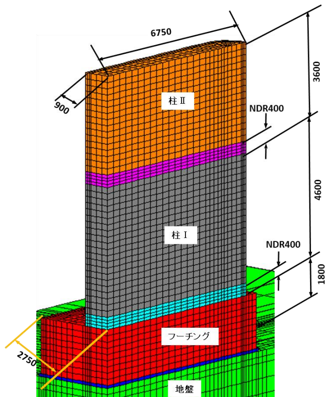
解析：1/4対象モデル
