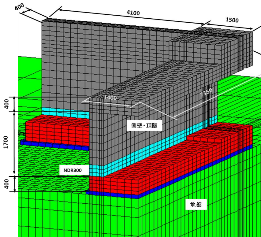
解析: 1/2対象モデル
