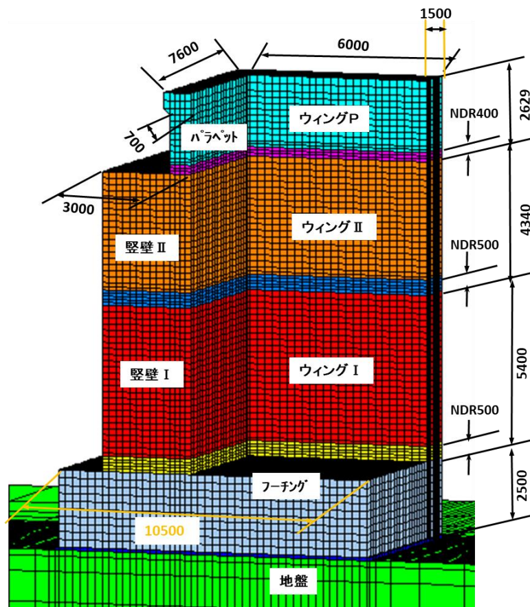
解析: 1/2対象モデル
