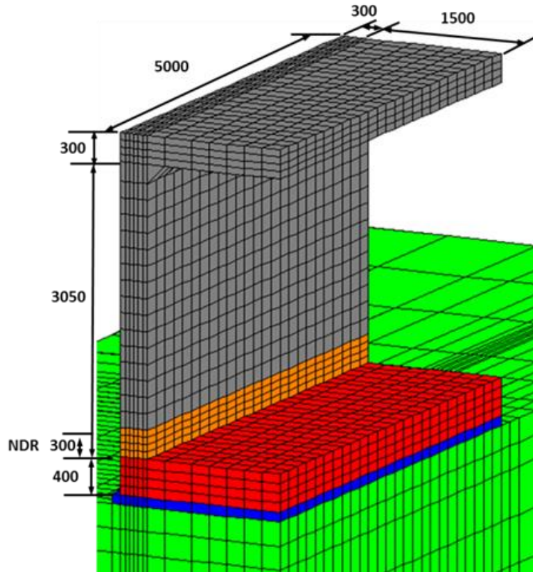
解析:1/4対象モデル
