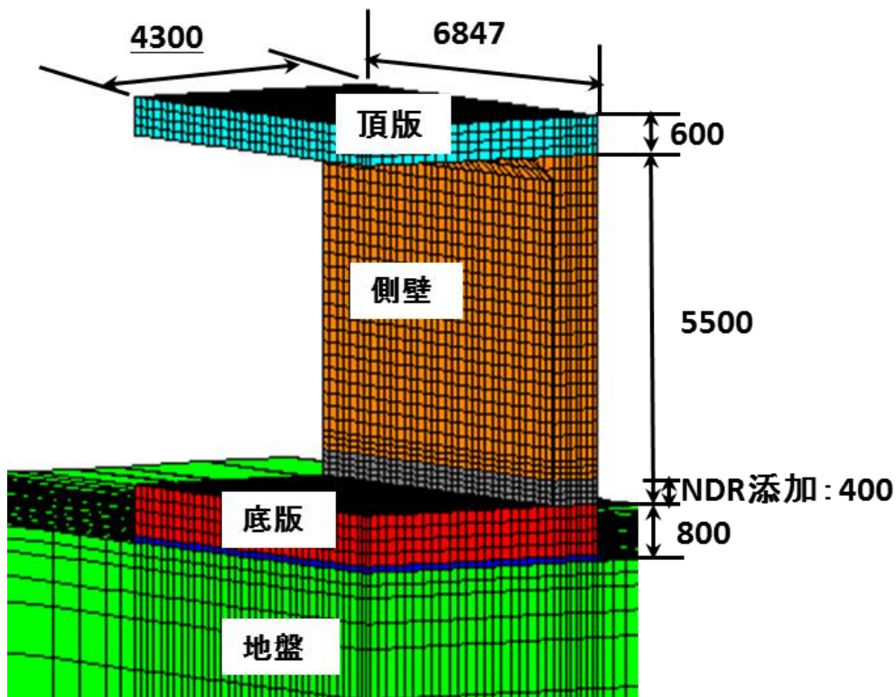
解析: 1/4対象モデル
