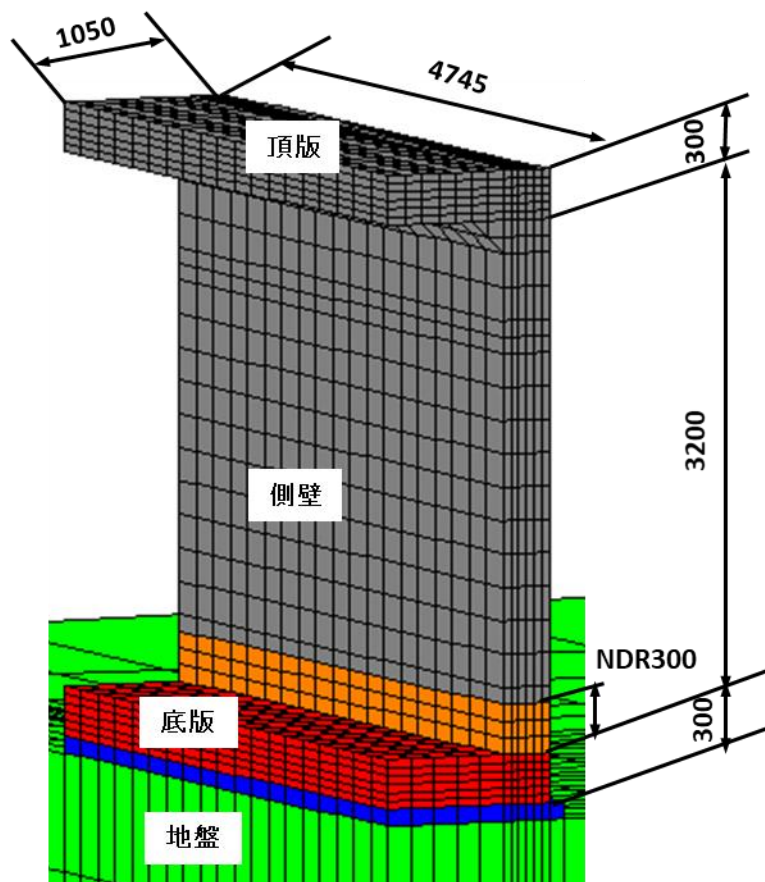
解析：1/4対象モデル
