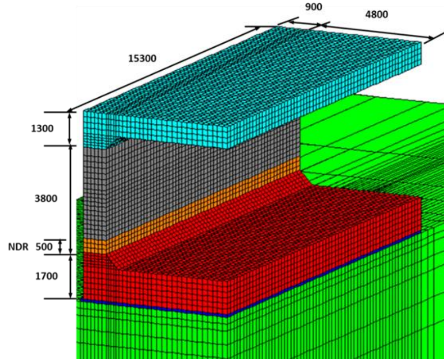
解析: 1/4対象モデル
