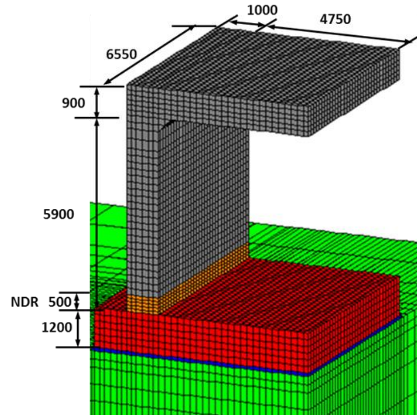
解析: 1/4対象モデル
